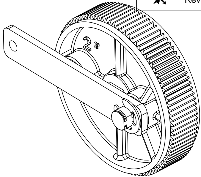
MONTAGE POUR 3900
