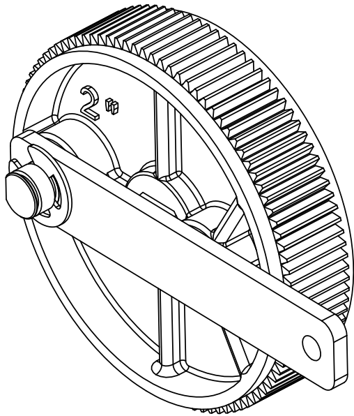
MONTAGE POUR 3150
