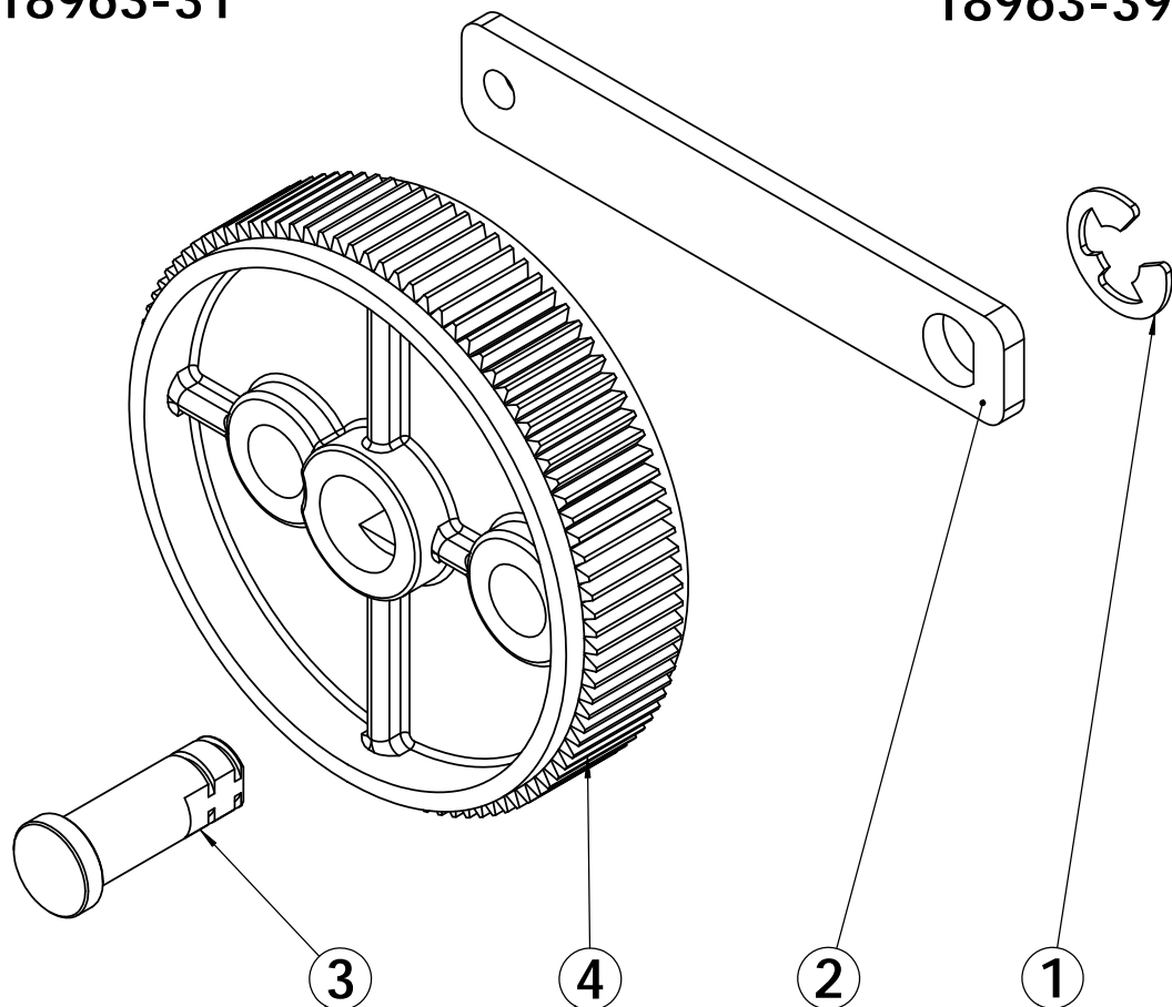
MONTAGE POUR 3150
